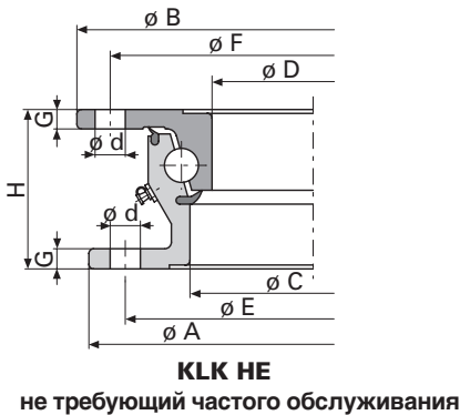
Схема сверления 1
